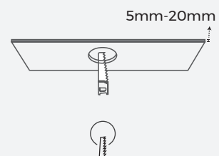
开孔尺寸: φ95mm
